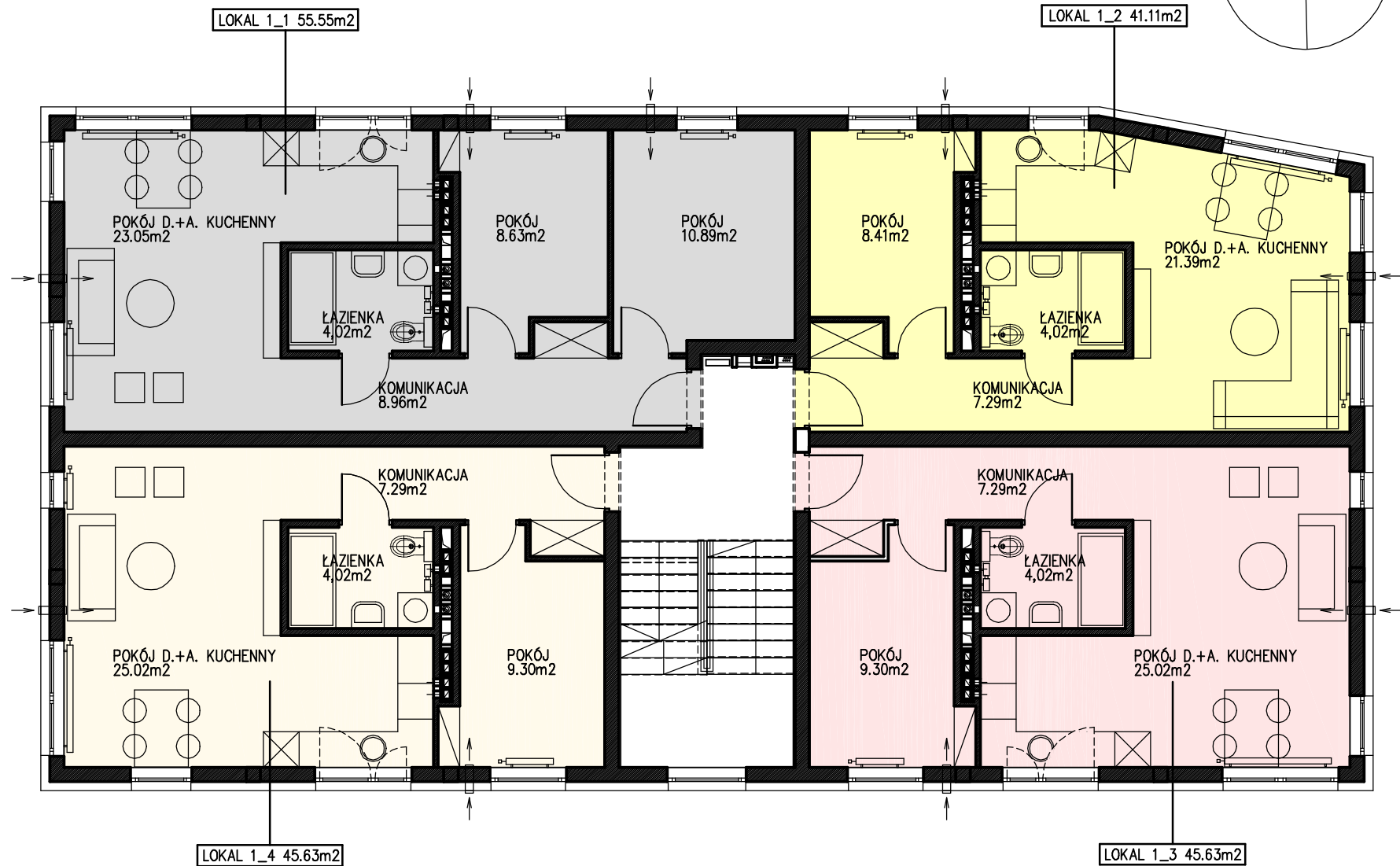
RZUT PIĘTRA 1
